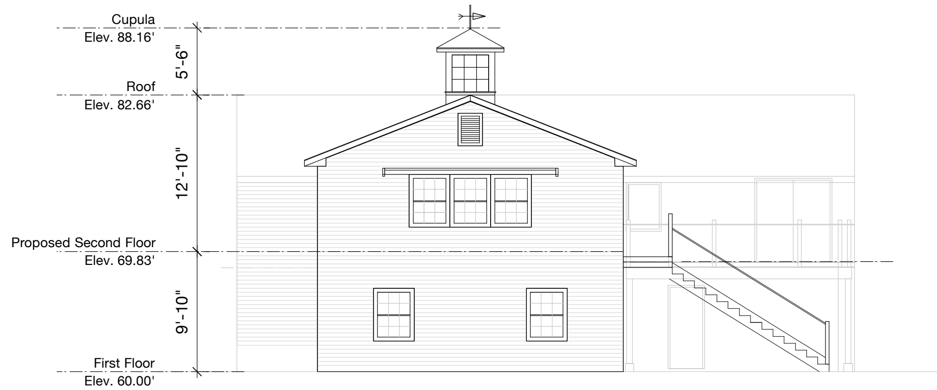
11 Side elevation Scale: 1/8" = 1'-0"
